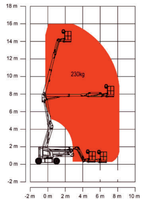
Bewegungsbereich PB DINO 16EZ-Li
