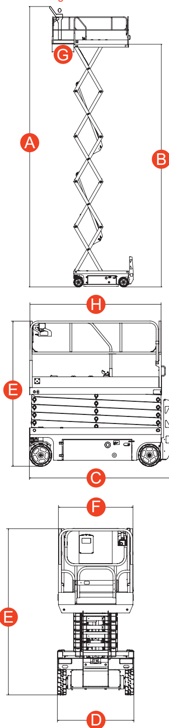
Abmessungen PB ECo S120-12EN
