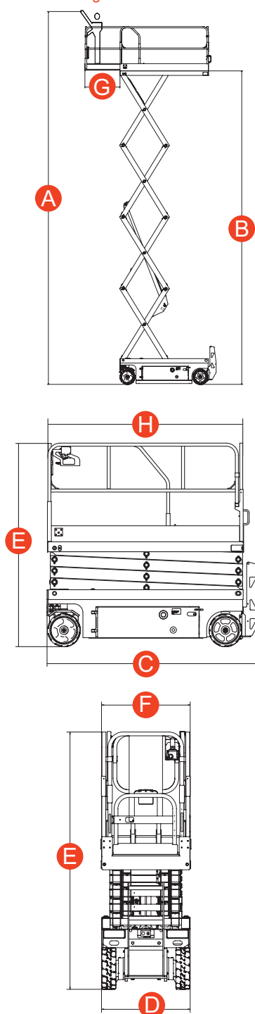
Abmessungen PB ECo S100-12EN
